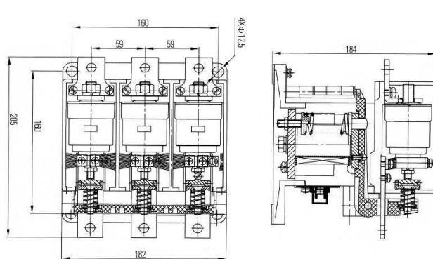
Рисунок 3. Габаритные размеры КВТ-1,14-250
