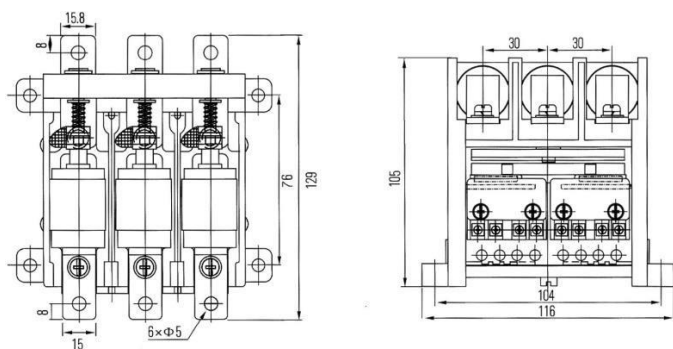
Рисунок 1. Габаритные размеры КВТ-1,14-63
