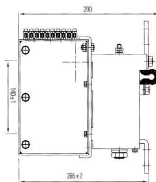
Рисунок 5. Габаритные размеры КВТ-1,14-630
