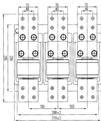
Рисунок 5. Габаритные размеры КВТ-1,14-630
