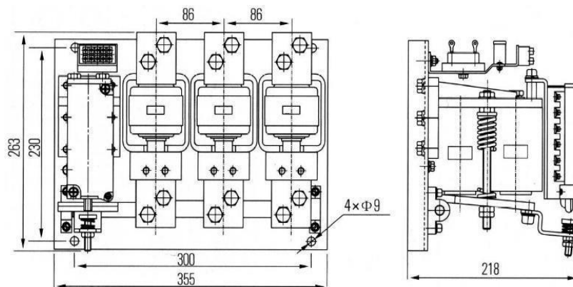
Рисунок 6. Габаритные размеры КВТ-1,14-1000/1250
